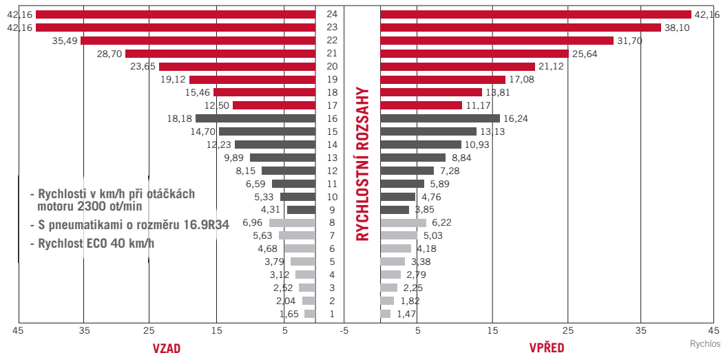
Diagram rychlostí převodovky 24x24 Hi-Lo 40 km/h
